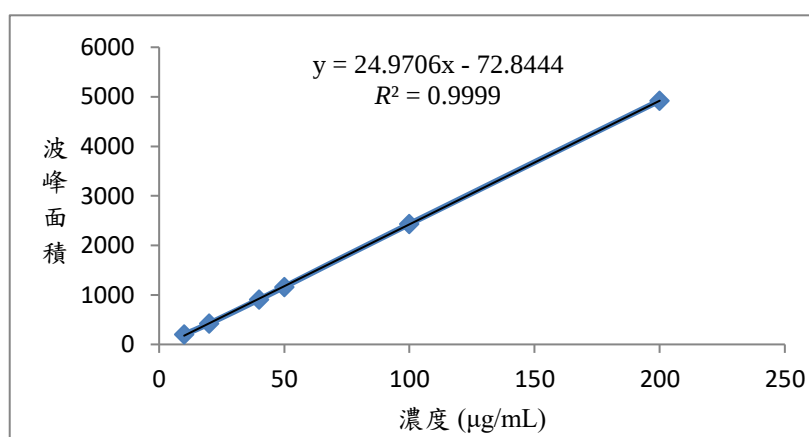
圖四、白花前胡甲素(Praeruptorin A)之檢量線圖
