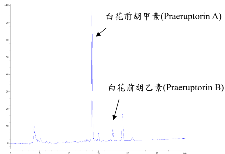
圖三、市售白花前胡檢品之 HPLC 層析圖
